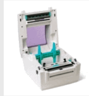
Gerät geöffnet
